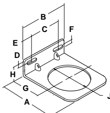
L-Fäste GPA-96-606
