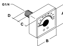
Manometer 18/28 Serie
