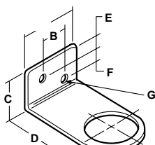
L-Fäste GRP-95-147
