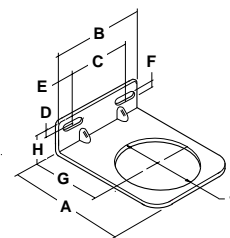
L-Fäste GPA-96-607
