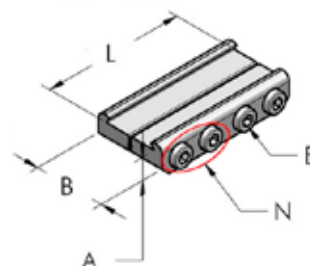
Förbindelsedon
